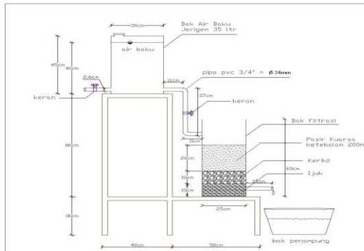
Gambar 1. Prototype Pengolahan Air Sederhana
