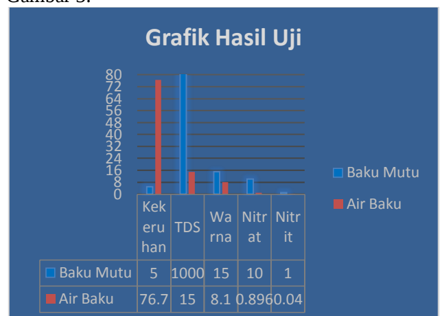
Gambar 3. Grafik hasil uji untuk air Sungai Batanghari pada Intake Pulau Pandan.
