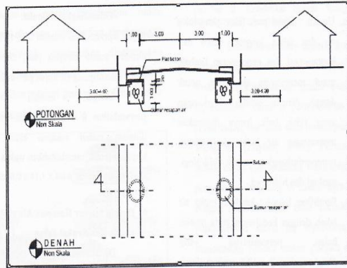
Gambar 4 : Resapan air pada Konstruksi Jalan
