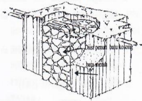
Gambar 2 : Konstruksi Sumur Resapan Air Isometri
