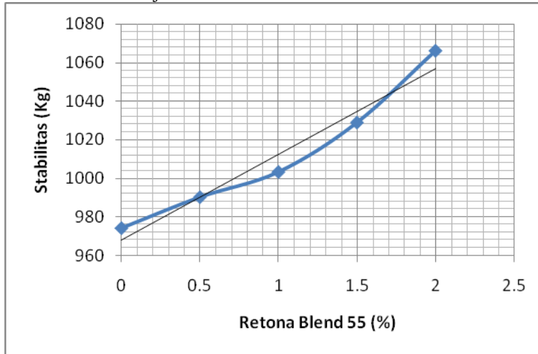
Gambar 4 Hubungan Kadar Retona Blend 55 dengan Stabilitas
