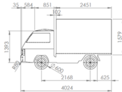
Gambar 2. Desain ukuran mobil box model X
