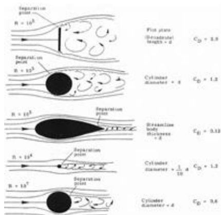
Gambar 1. Hubungan Antara Drag Koefisien dan Variasi Bentuk
