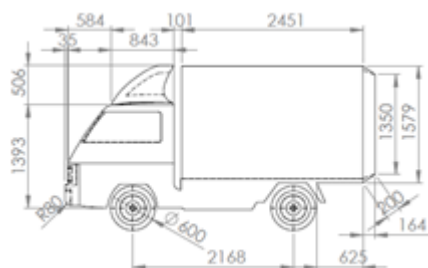
Gambar 4. Desain ukuran mobil box model Y
