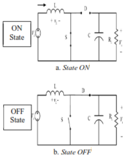
Gambar 5 Rangkaian boost pada saat a.state ON dan b. state OFF
