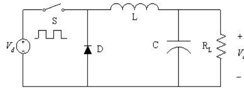
Gambar 3 Rangkaian buck converter kondisi saklar terbuka
