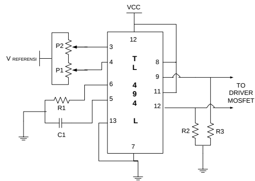
Gambar 12 Rangkaian Pembangkitan Sinyal PWM
