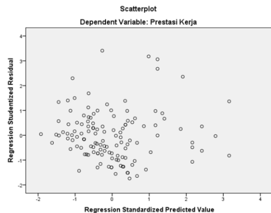
Gambar 1 Uji Heteroskedastisitas
