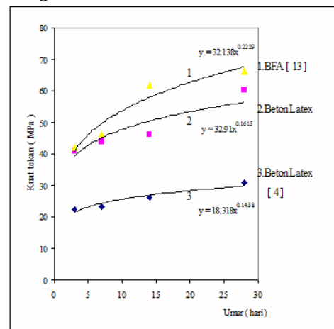
Grafik 1. Hubungan antara umur dan kekuatan beton.
