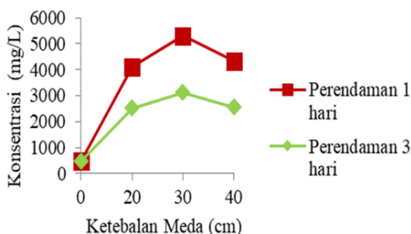
Gambar 2 Pengaruh Media Filter Batang Pisang Terhadap Parameter COD
