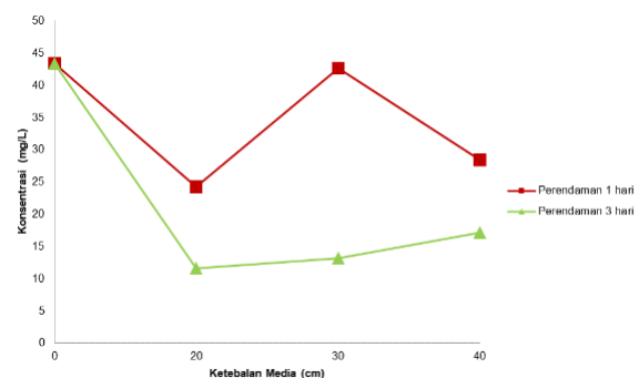
Gambar 4 Pengaruh Media Filter Batang Pisang Terhadap Parameter MBAS
