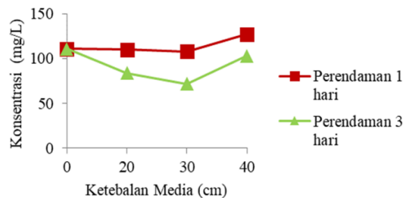
Gambar 3 Pengaruh Media Filter Batang Pisang Terhadap Parameter TSS
