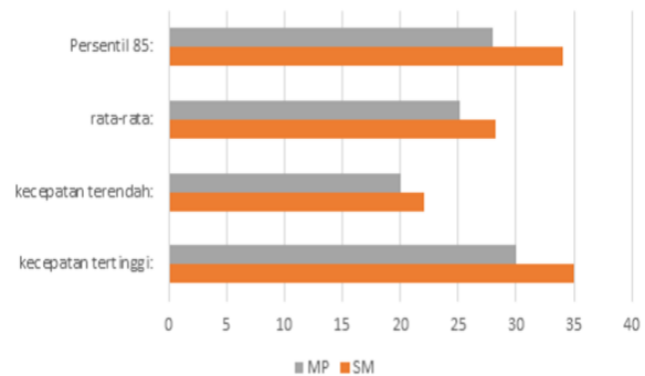
Gambar 9 Grafik arah timur Jalan Raya Kepandean
