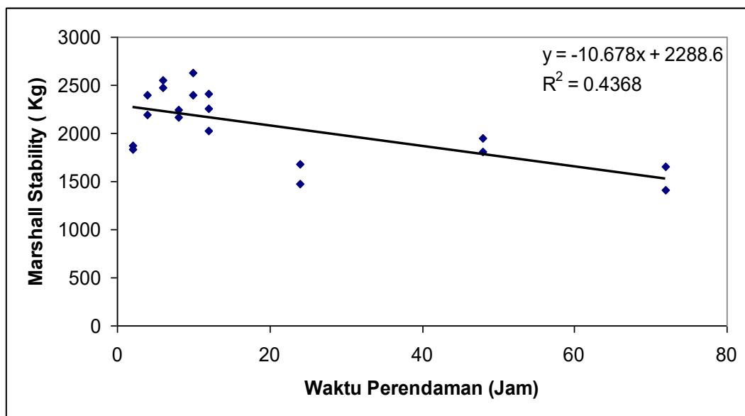
Gambar 1. Grafik Hubungan Waktu Perendaman dengan Stabilitas Marshall
